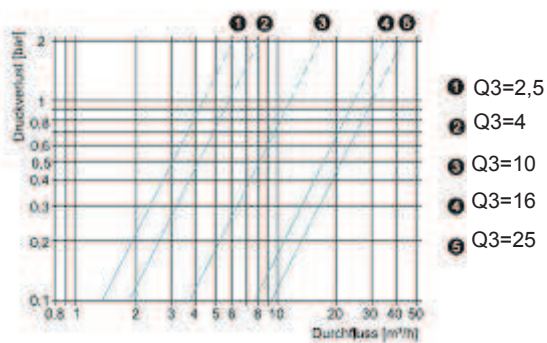
Druckverlustkurve
