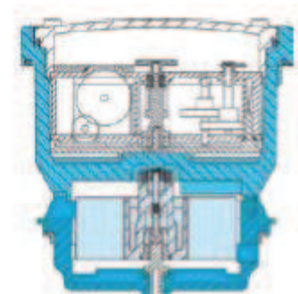
Schnittzeichnung MTK
