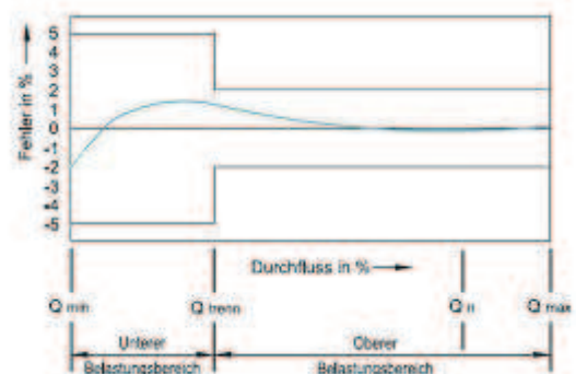
Typische Fehlerkurve
