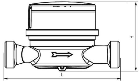
Maßzeichnungen Einstrahlzähler Standard und Modularis
