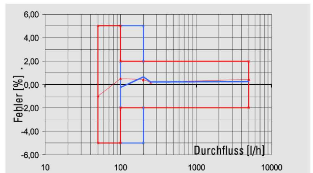
Typische Fehlerkurve Klasse C und Klasse B
