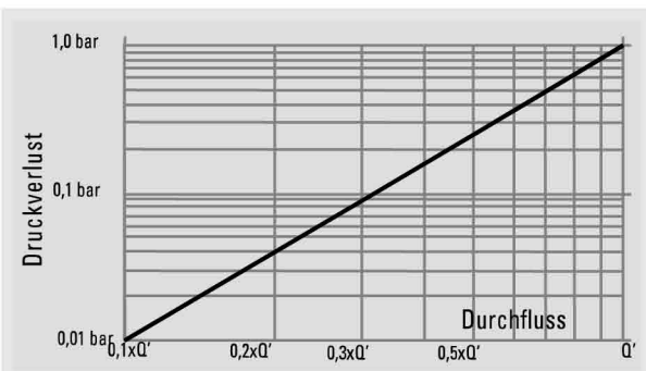
Druckverlustkurve
