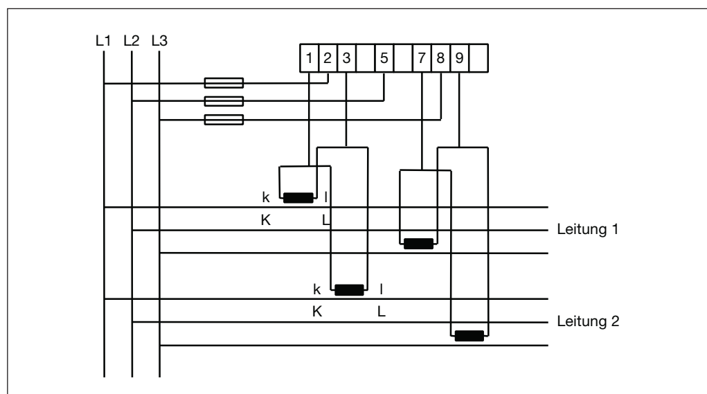
Abb. 8-3: Energiesummierung
