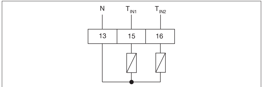
Abb. 8-4: Tarifeingänge, Anschlussbild
