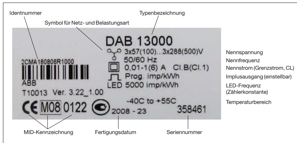
Abb. 3-2: Geräteetikett
