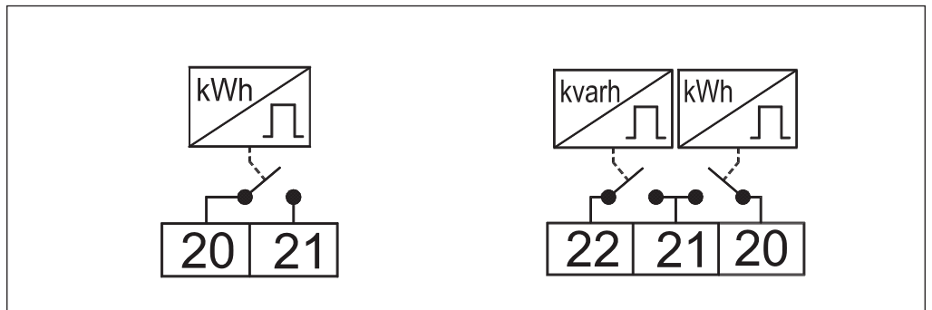
Abb. 8-5: Impulsausgänge, Anschlussbild
