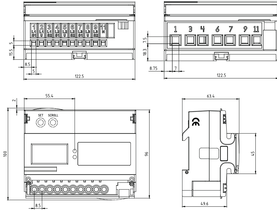
Wandlerzähler
