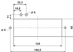
Abdeckung lang
